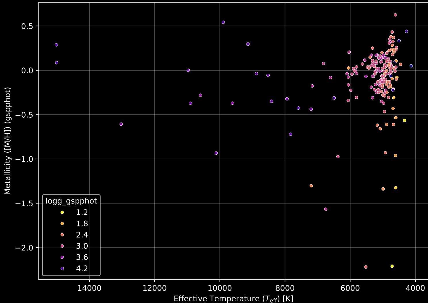
APOGEE DR17 Field: [128+04] Stellar Population Parameters (n= 206)
